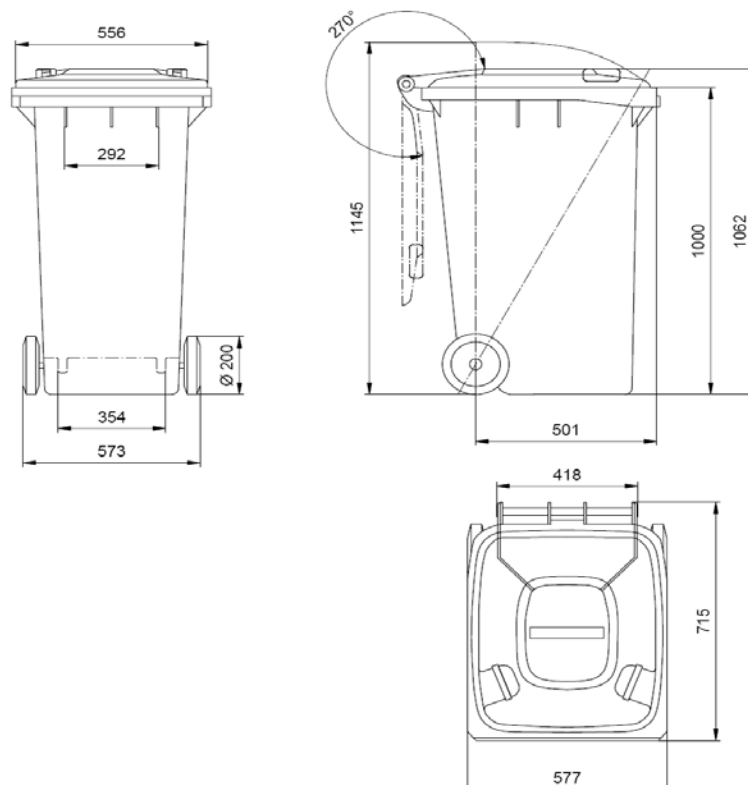
Dibujo acotado (medidas en mm.)
